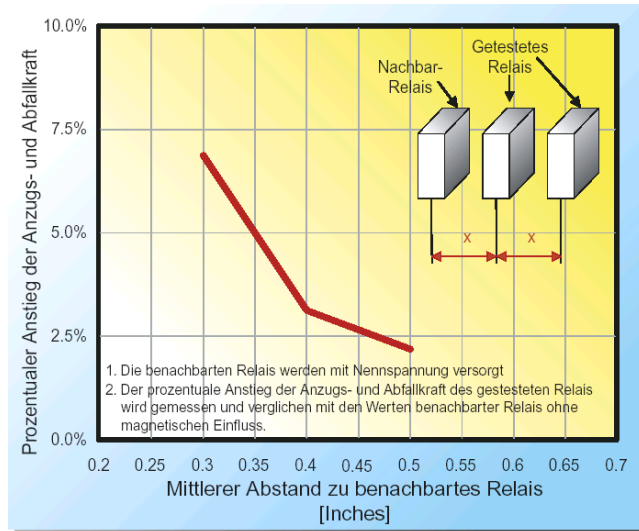
Abbildung 3: EMR Abstandsanforderungen
