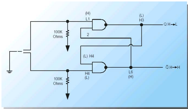
Abbildung 5: Schaltung zur Kontakt-Entprellung
