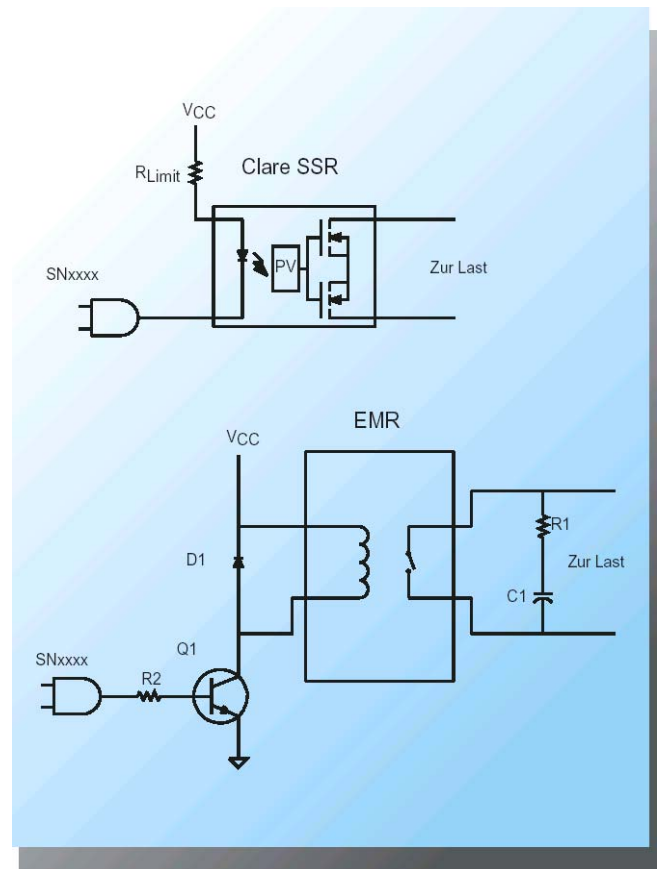
Abbildung 6: SSR und EMR Ansteuervergleich
