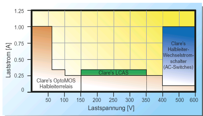
Abbildung 1: CLARE Halbleiterrelais (SSRs)
