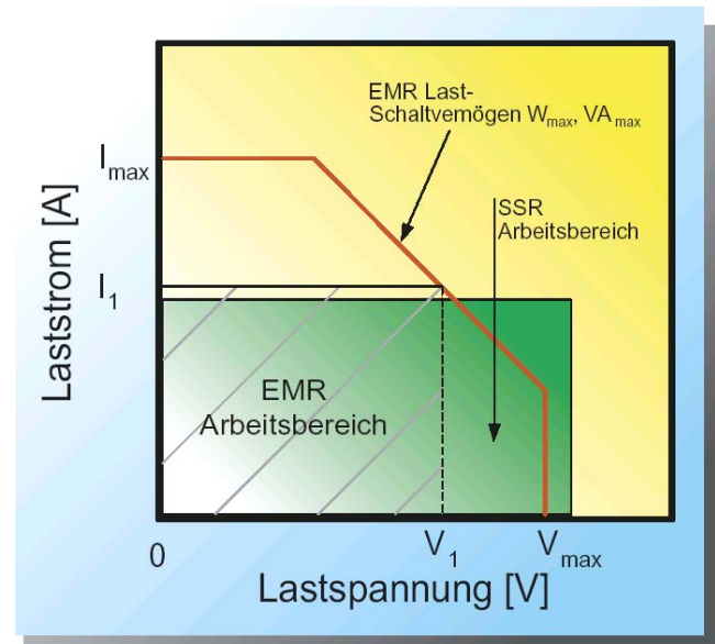
Abbildung 2: Diagramm zur Abnahme des Schaltvermögens
